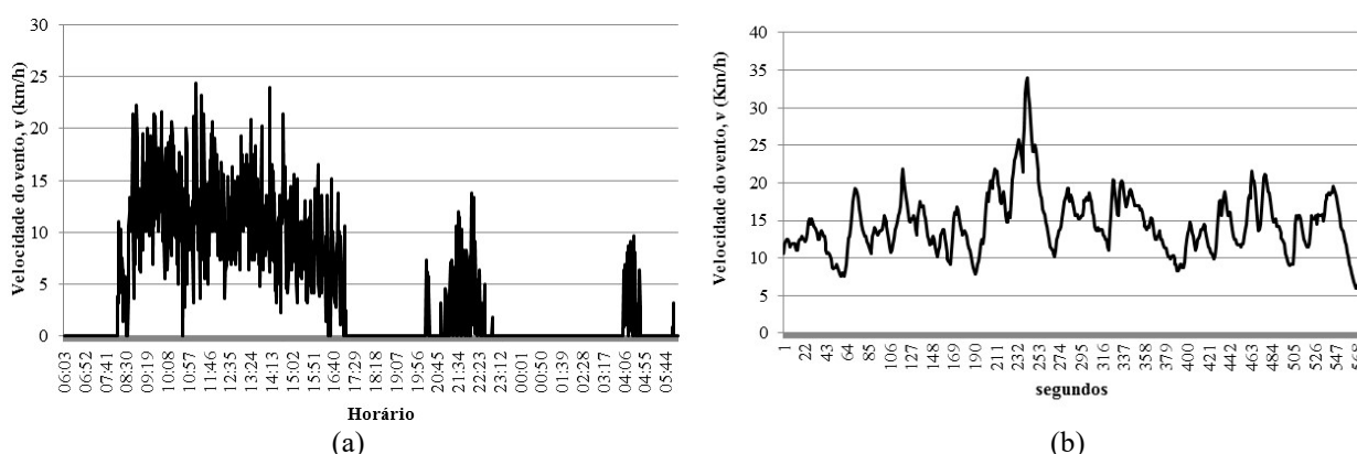
Figura 10 – Velocidade do vento: (a) período de 24h (b) período de 10 minutos.
