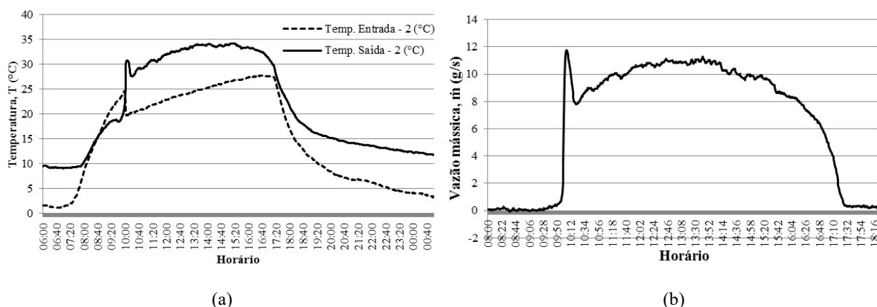
Figura 9 - (a) Curva de temperatura de entrada e saída do coletor (b) curva de vazão mássica da água.
