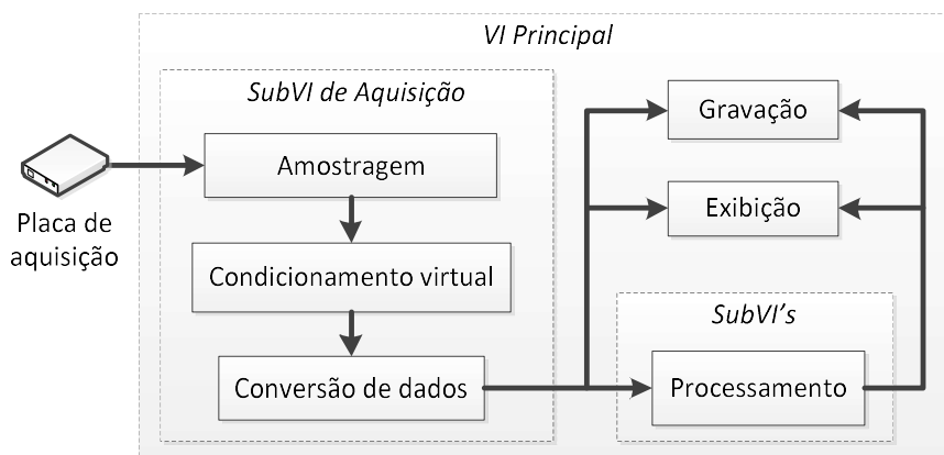
Figura 5 – Diagrama de blocos do programa de monitoramento DAQSOL.
