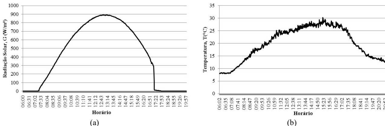
Figura 8 - (a) Curva de radiação solar (b) curva de temperatura ambiente
