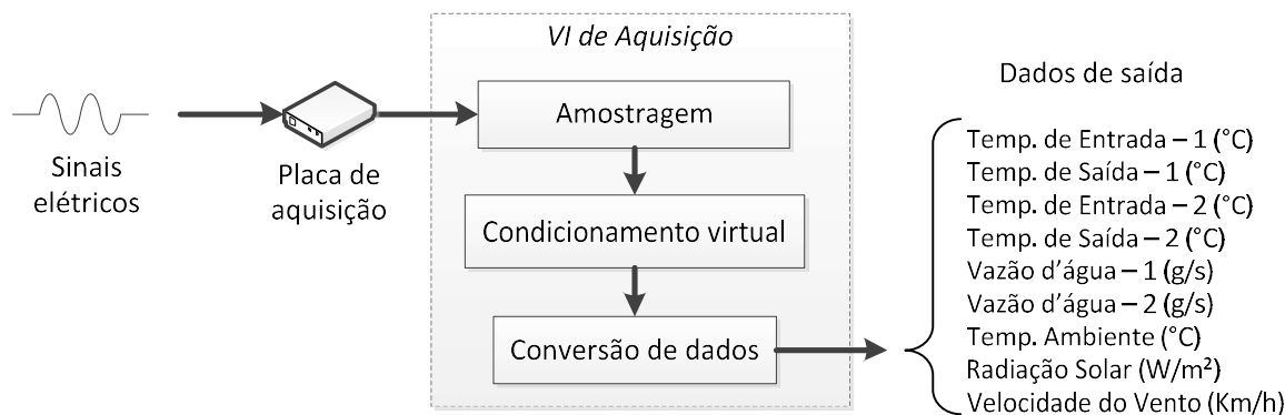
Figura 4 – Diagrama funcional para obtenção das informações de interesse.
