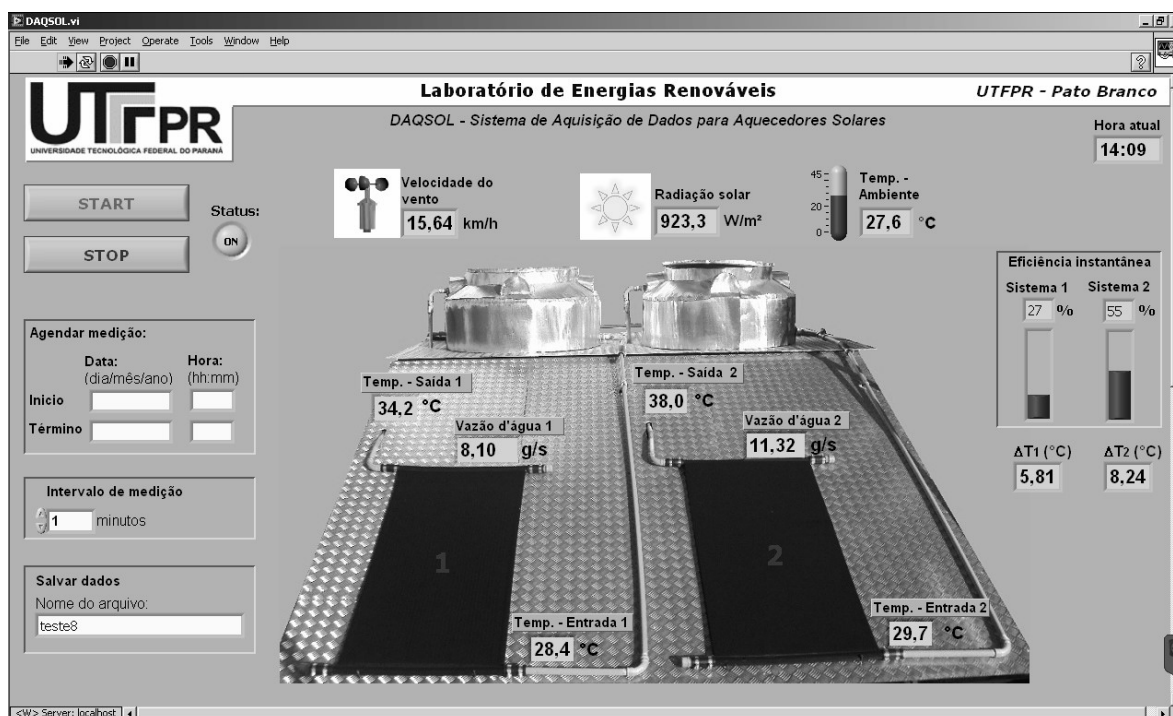
Figura 6 – Tela principal do aplicativo DAQSOL desenvolvido.
