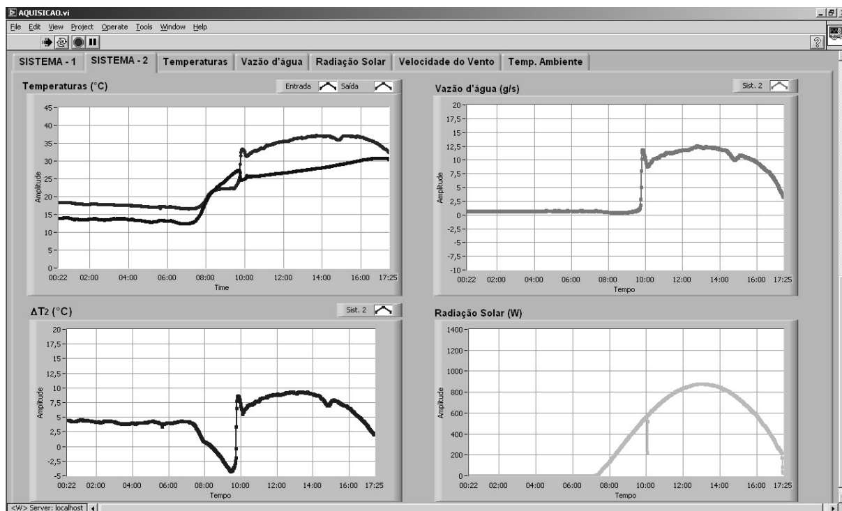
Figura 7 – Tela secundária do aplicativo desenvolvido. Gráficos com as informações atualizadas em tempo real.
