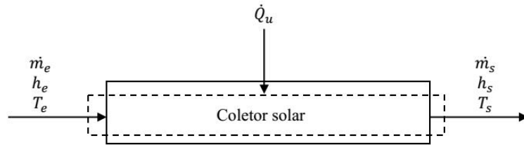
Figura 1- Representação de um coletor solar plano e grandezas envolvidas.
