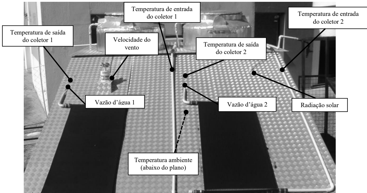
Figura 3 – Arranjo experimental do Laboratório de Energias Renováveis da UTFPR.
