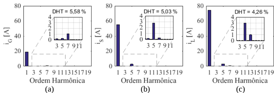
Figura 7 – Espectro das correntes (a) da rede, (b) do inversor e (c) da carga no tempo de dois segundos.
