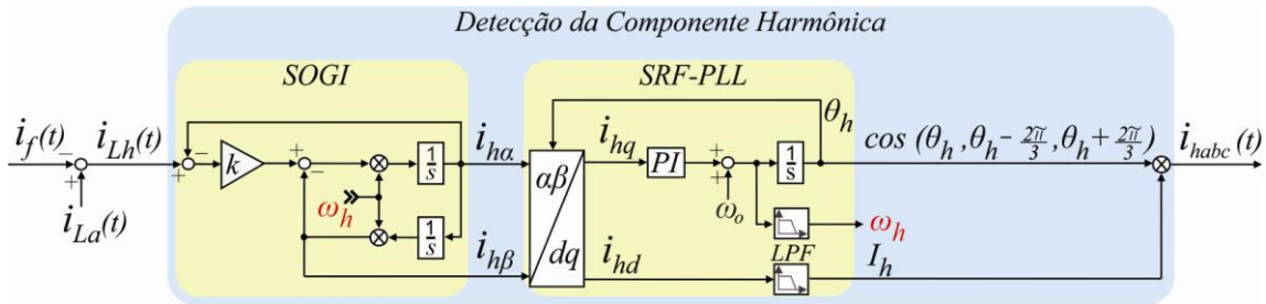
Figura 4 – Método de detecção da componente harmônica de maior amplitude.
