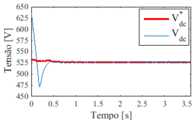
Figura 5 – Controle da tensão do barramento cc.
